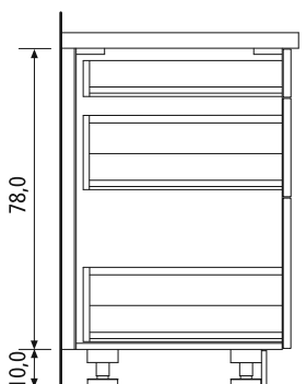
C2 78 Kasten in korpushoogte 78 cm Keukens met grepen
